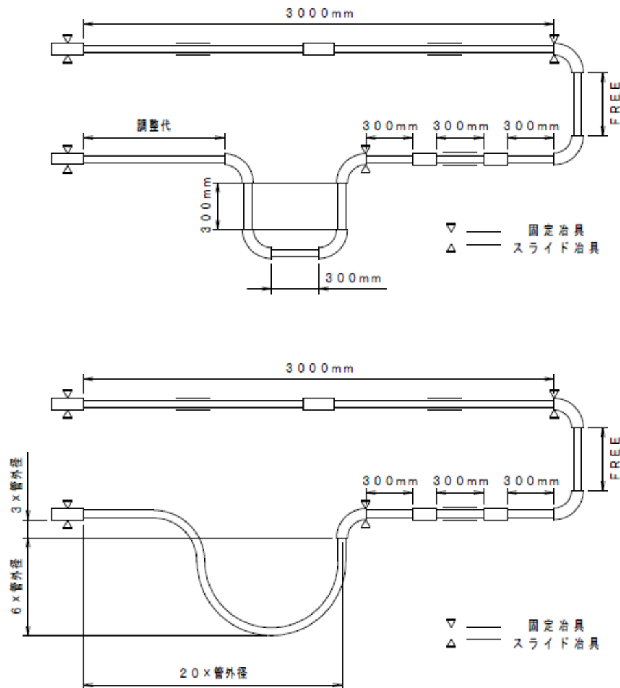
8 試験配管例
