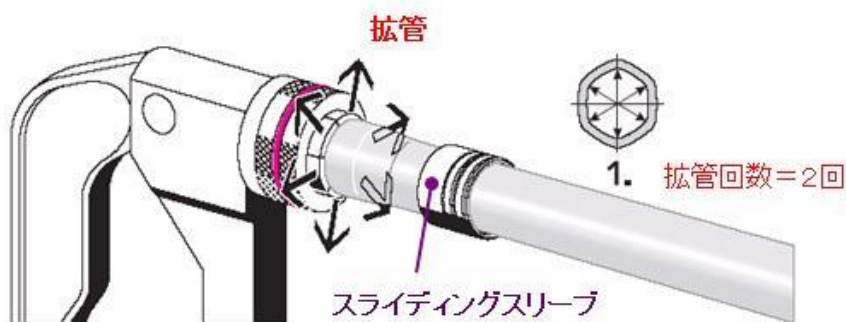
拡管作業（例）
