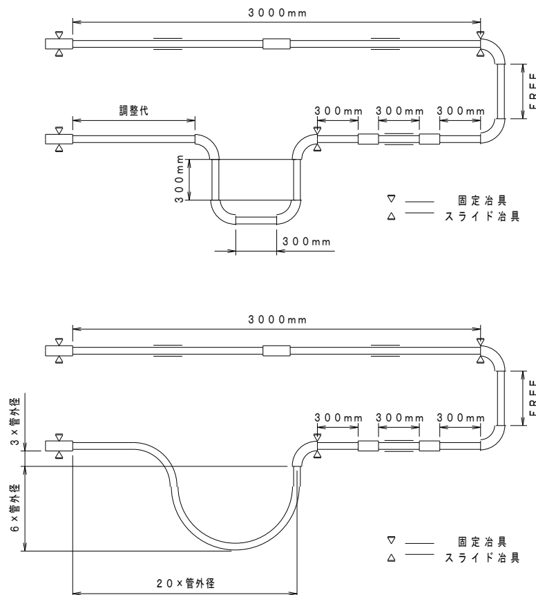
図 4 試験配管例
