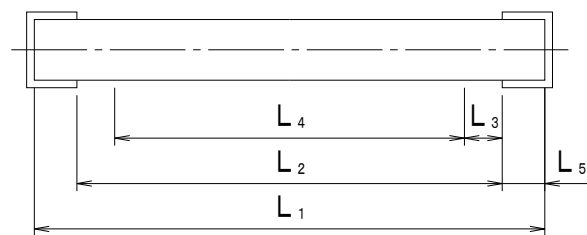
図 1 試験片長さ
