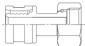
d) 管をスリーブで締め付けて、水密性を確保する継手
