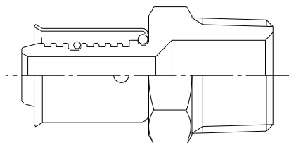
a) 管をスリーブで加締めて水密性を確保する継手
