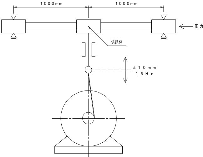
図 5 たわみ試験装置
